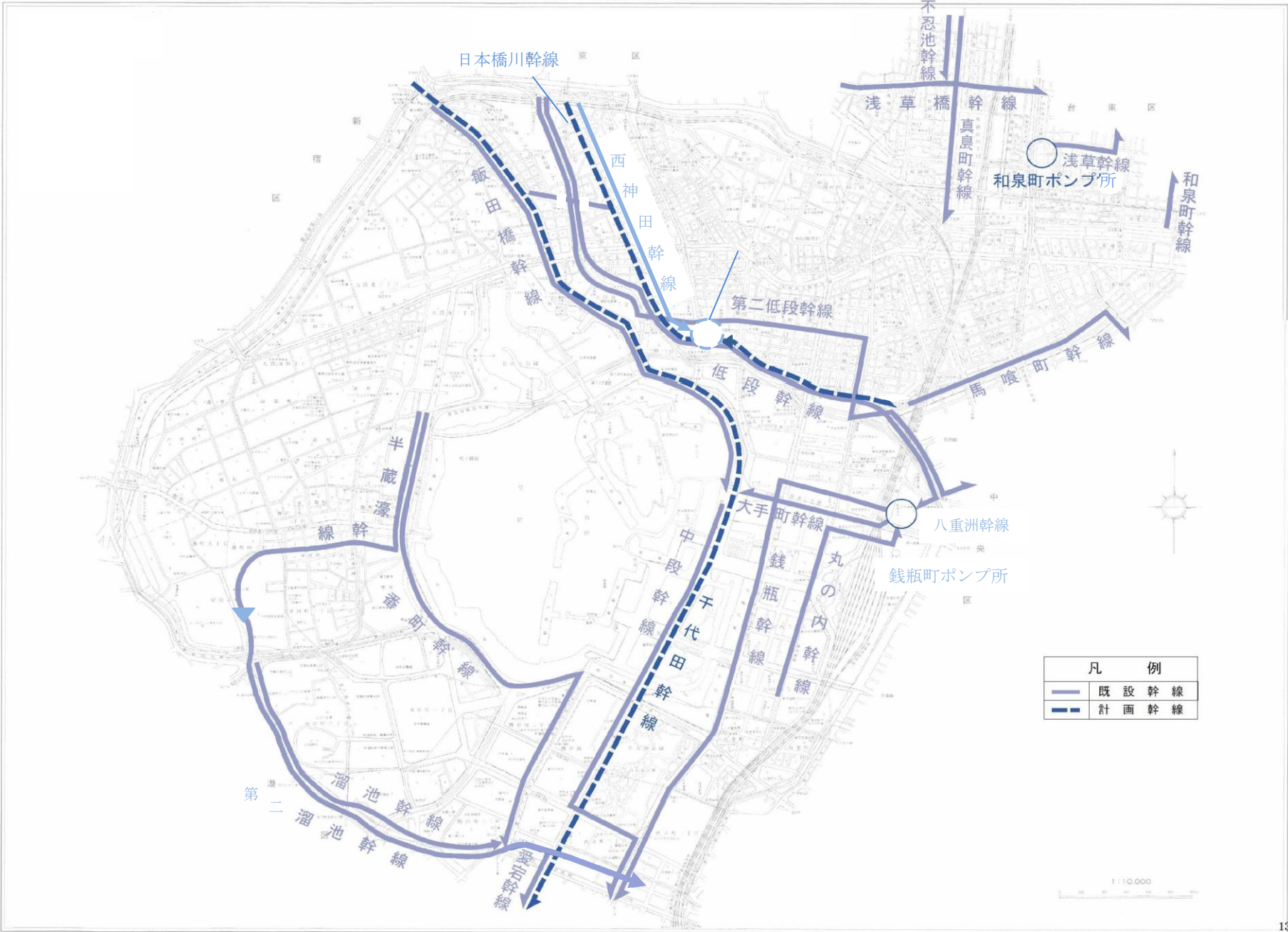
下水道幹線の計画図（下水道局中部下水道事務所）
