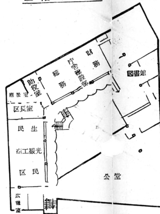
二階平面図
