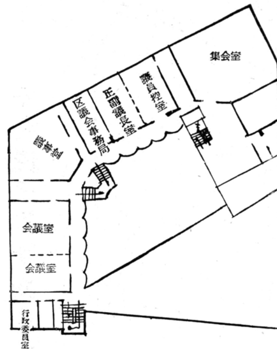
四階平面図
