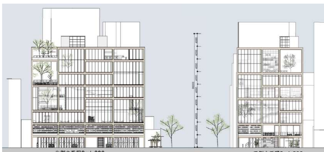
図 26 神保町交差点に面した街区の共同建て替えのモデルスタディの立面図
