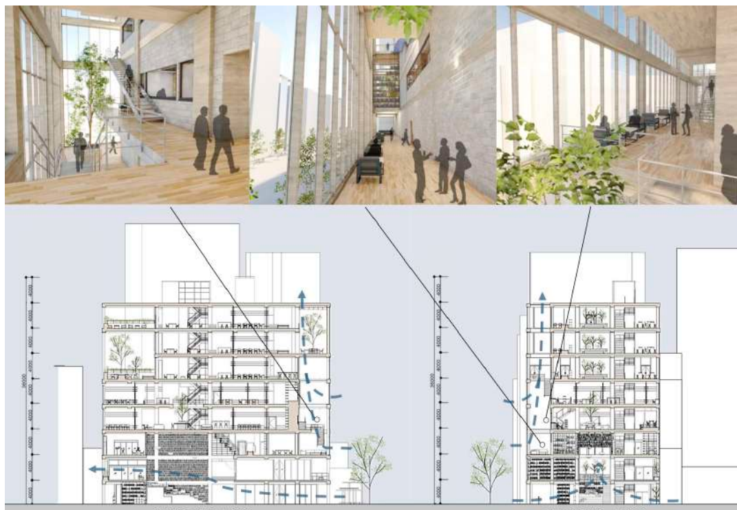
図 27 神保町交差点に面した街区の共同建て替えのモデルスタディの断面図
