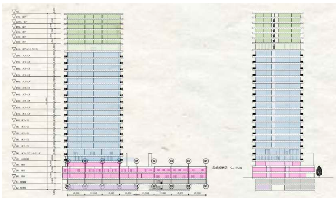
図 14 神保町交差点に面した市街地再開発のモデルスタディの立面図
