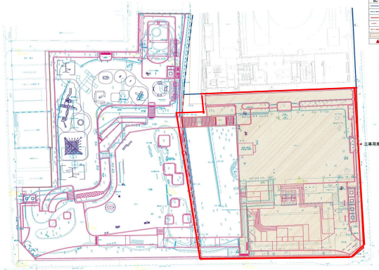
施工展開図① 第一期 [H29. 10～H30. 8]
