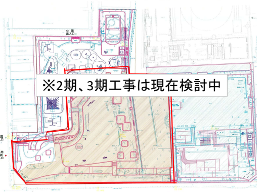
施工展開図② 第二期 [H30. 10～H31. 3]
