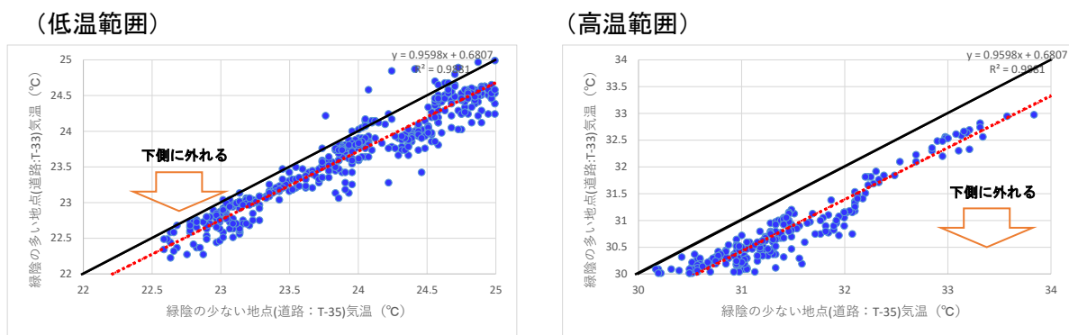
図 5-33 緑陰多(T-33)・緑陰少(T-35)の気温比較の低温・高温範囲拡大図(夜間)
