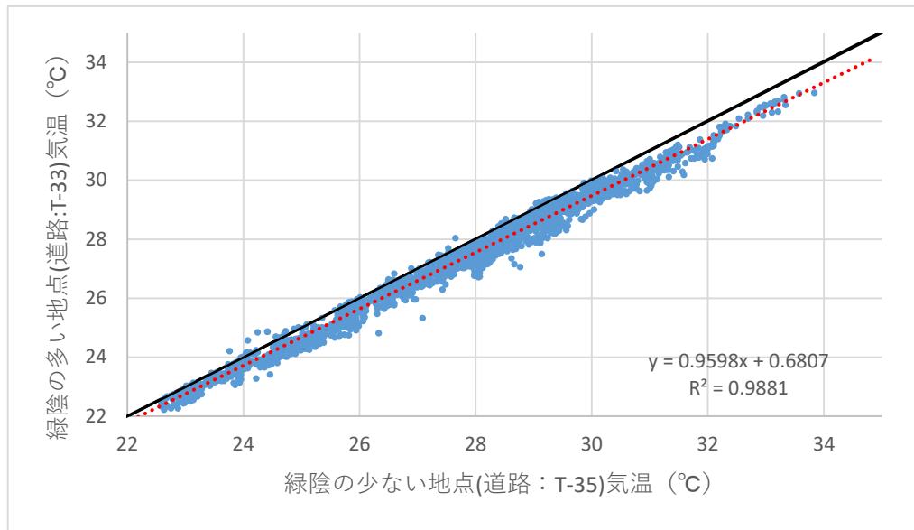
図 5-32 緑陰多地点(T-33：道路環境)と少地点(T-35：道路環境)の気温比較図(夜間)
