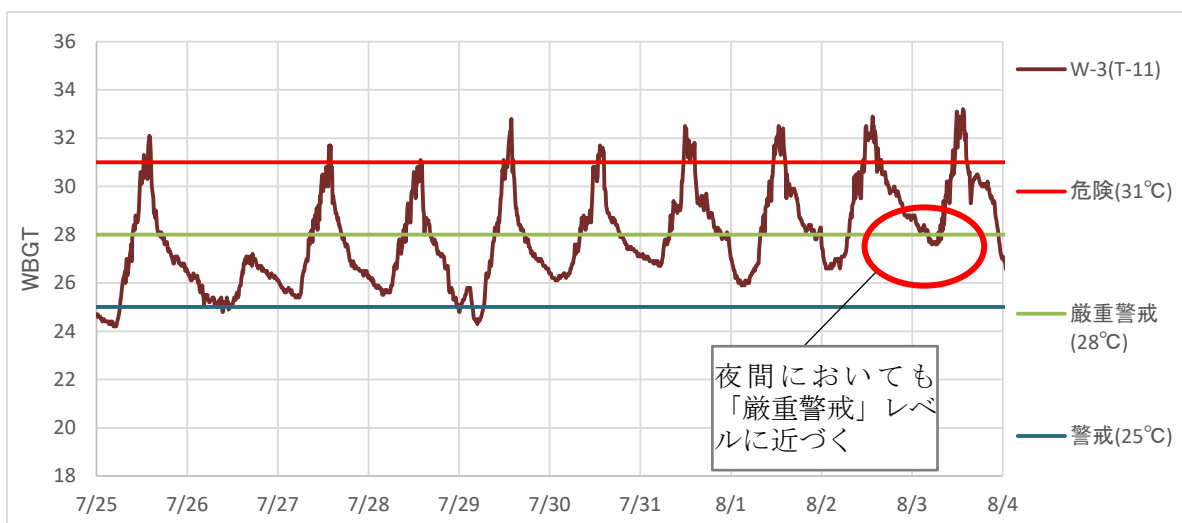
図 5-41 都市環境(神田駅前)W-3(T-11) 地点の暑さ指数(WBGT)観測結果
