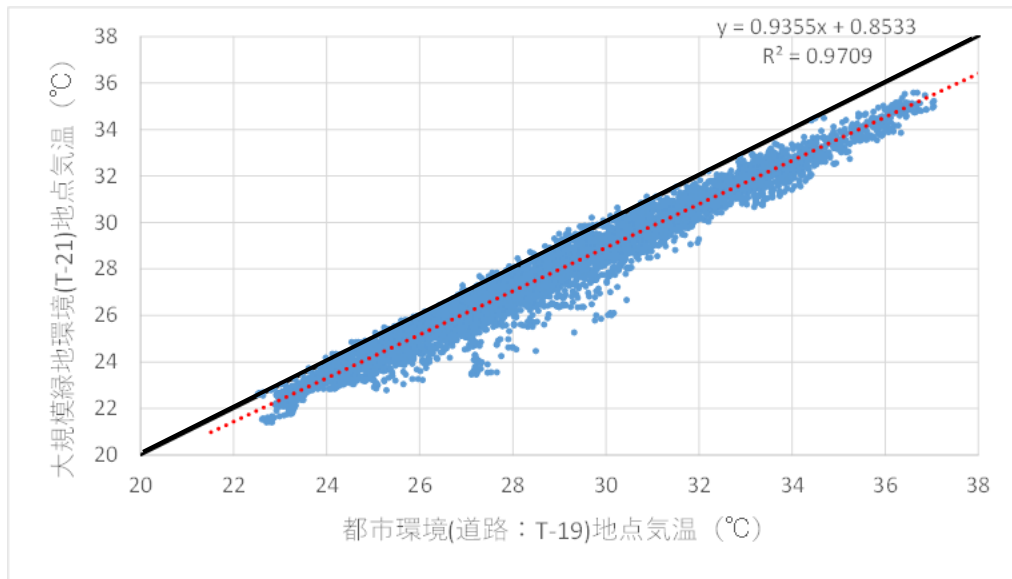
図 5-25 大規模緑地環境（北の丸公園：T-21）と都市環境（住宅地：T-19）の気温比較図
