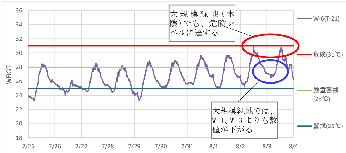
図 5-43 大規模緑地 W-6(T-21) 地点の暑さ指数(WBGT) 観測結果
