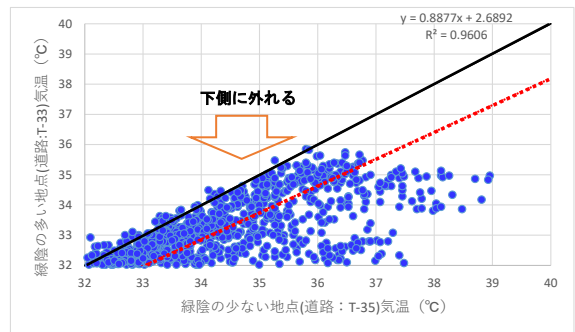
図 5-31 緑陰多 (T-33) ・ 緑陰少 (T-35) の気温比較の低温 ・ 高温範囲拡大図
