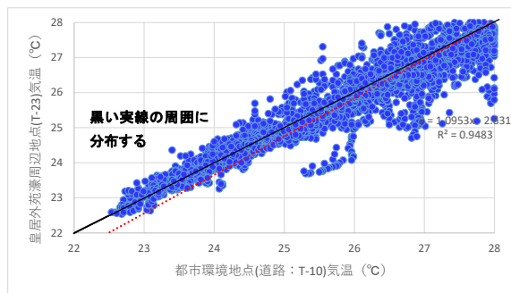
図 5-36 T-23・T-10 の気温比較の低温・高温範囲拡大図
