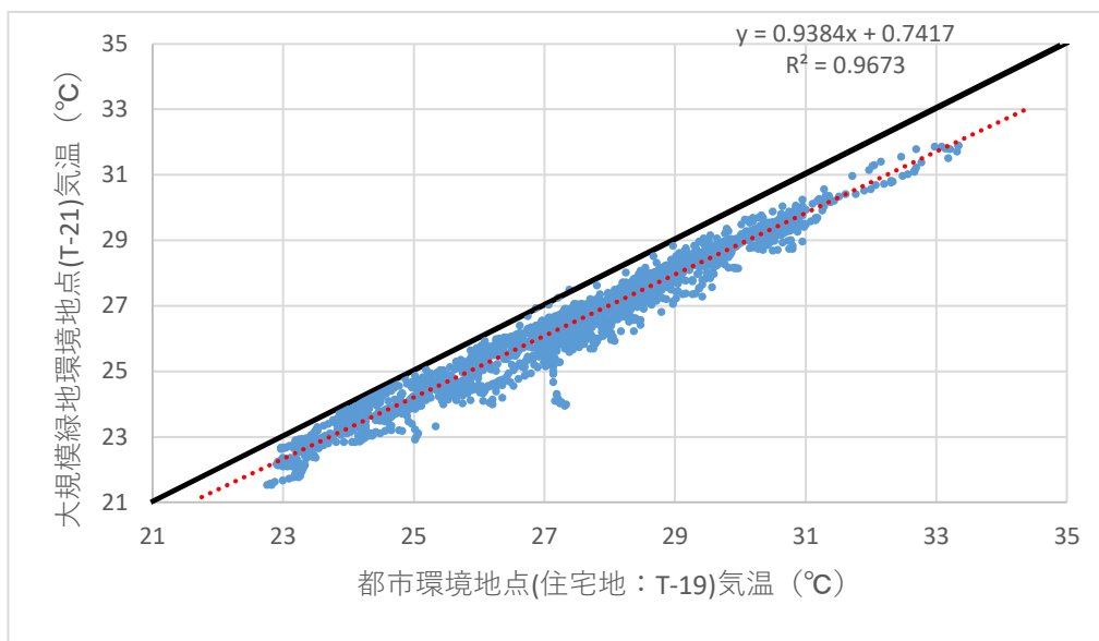
図 5-27 大規模緑地環境(T-21)と都市環境(住宅地：T-19)の気温比較図（夜間）
