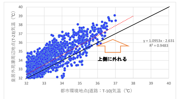
図 5-36 T-23・T-10 の気温比較の低温・高温範囲拡大図
