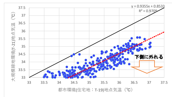
図 5-26 大規模緑地環境（T-21）と都市環境（T-19）との気温比較の低温・高温範囲拡大図
