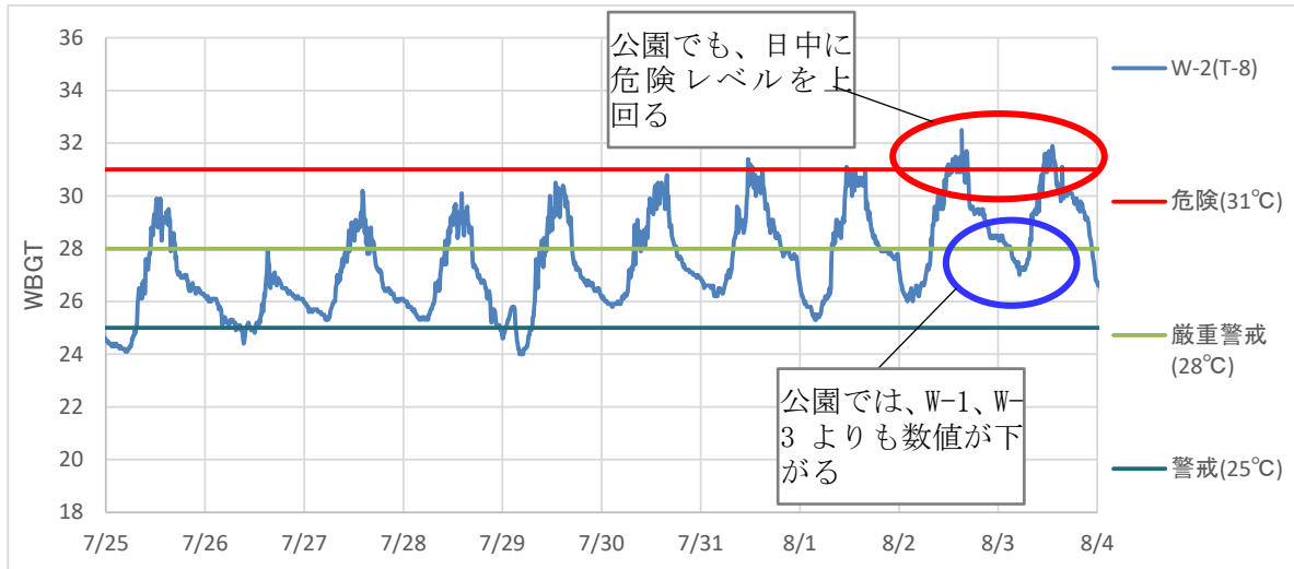
図 5-42 公園環境 W-2(T-8) 地点の暑さ指数(WBGT) 観測結果
