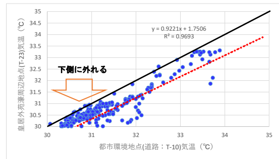
図 5-38 T-23・T-10 の気温比較の低温・高温範囲拡大図(夜間)
