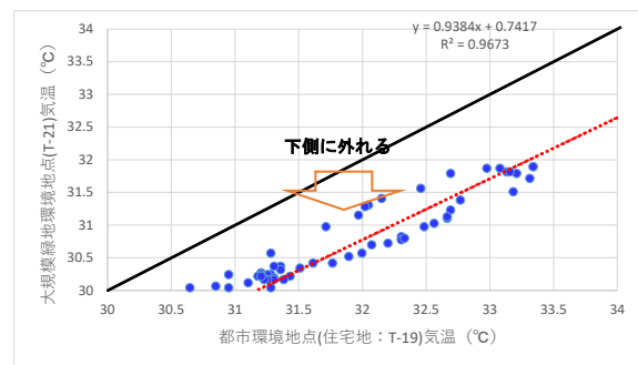
図 5-28 大規模緑地環境(T-21)と都市環境(T-19)の気温比較の低温・高温範囲拡大図(夜間)
