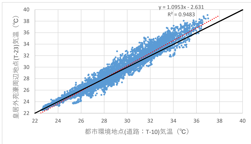
図 5-35 皇居外苑濠周辺地点(T-23)と道路環境地点(T-10)の気温比較図
