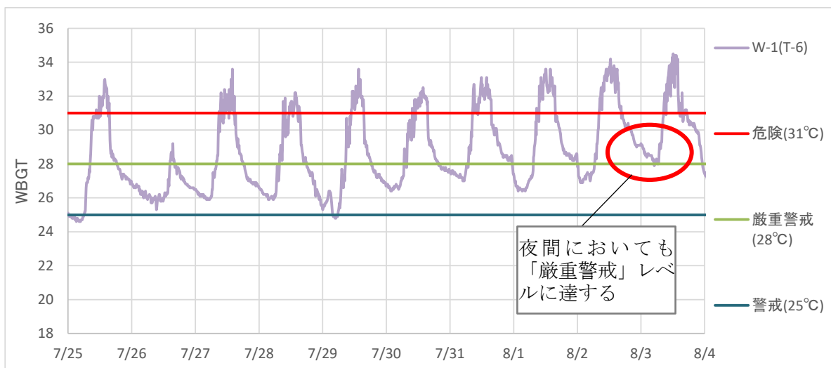
図 5-40 都市環境(オフィス・住宅地)W-1(T-6) 地点の暑さ指数(WBGT)観測結果
