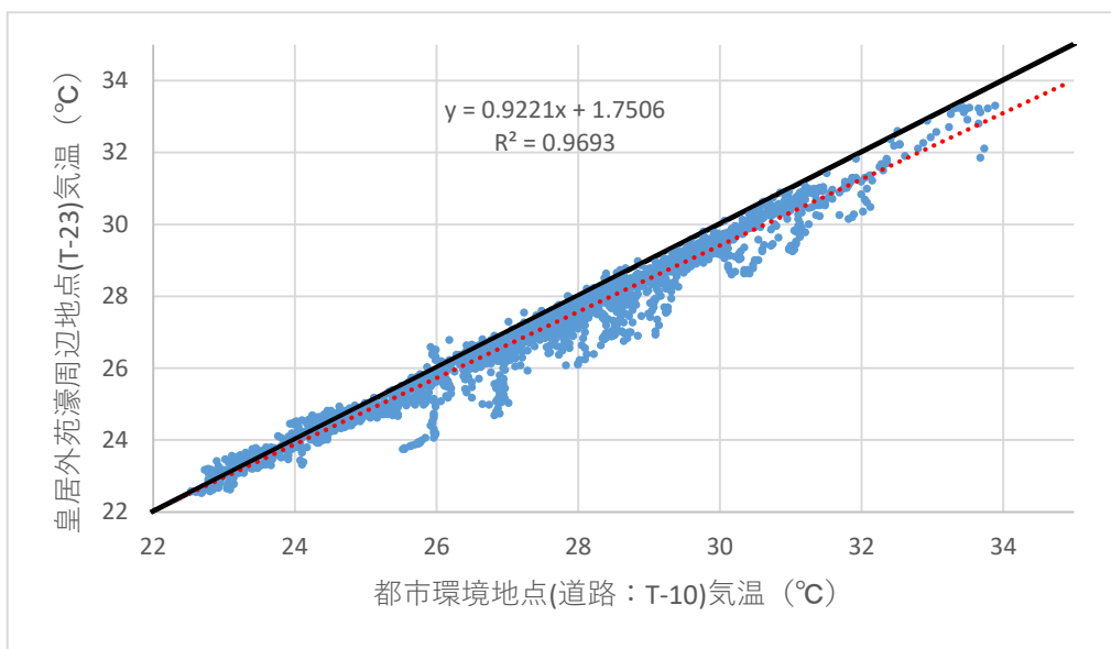
図 5-37 皇居外苑濠周辺地点(T-23)と都市環境地点(道路：T-10)の気温比較図(夜間)
