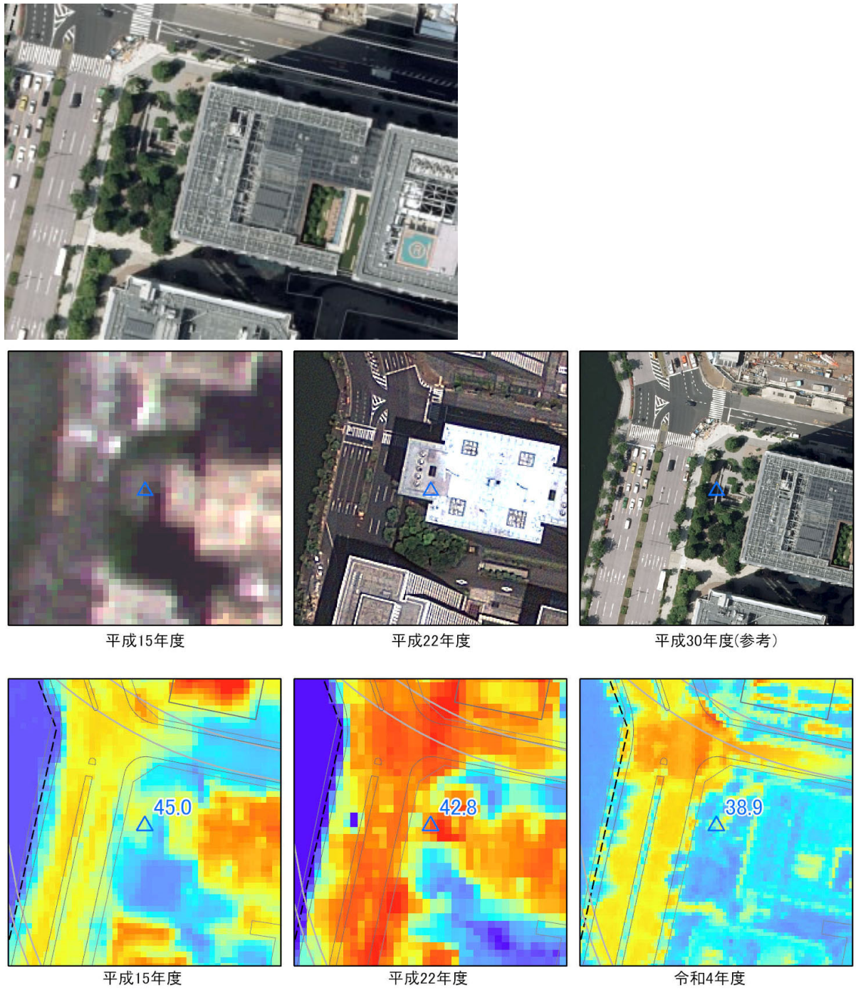
図 6-6 (9) ヒートアイランド対策実施箇所検証点の温度比較
