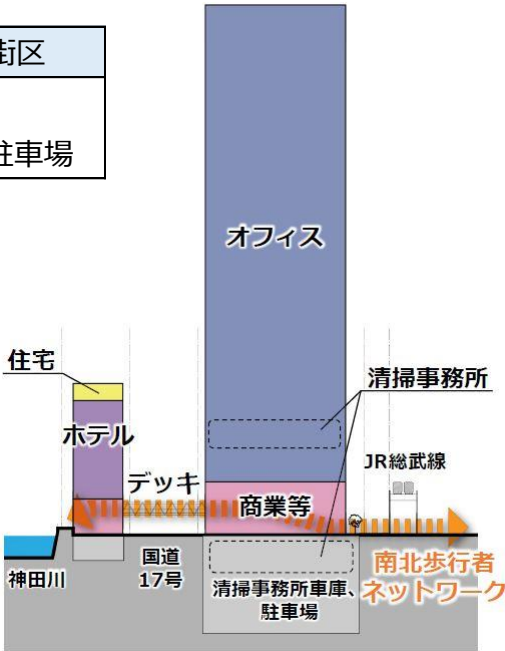
【南北断面イメージ】
