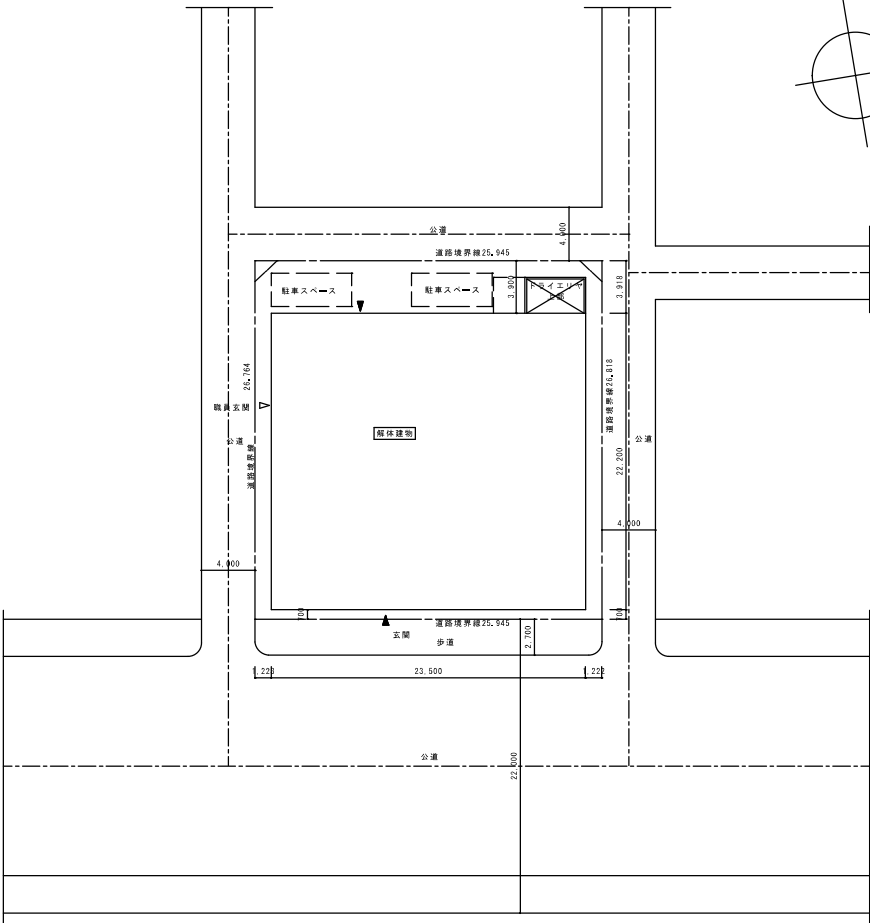
配置図 1/200
