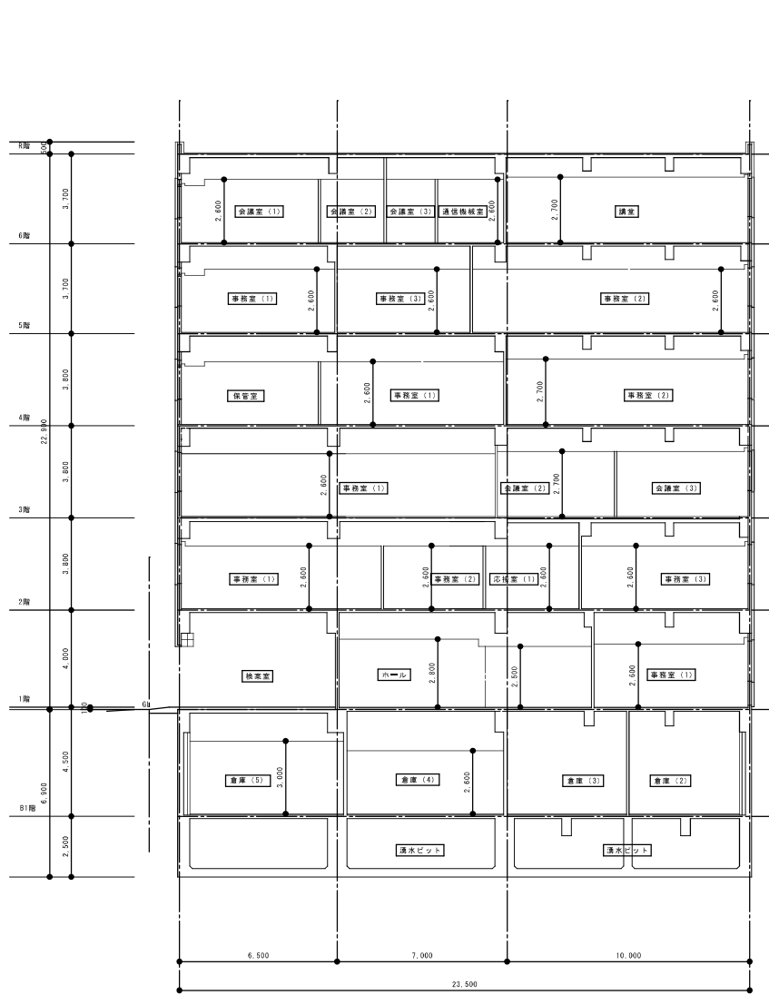
西一東断面図 1/200
