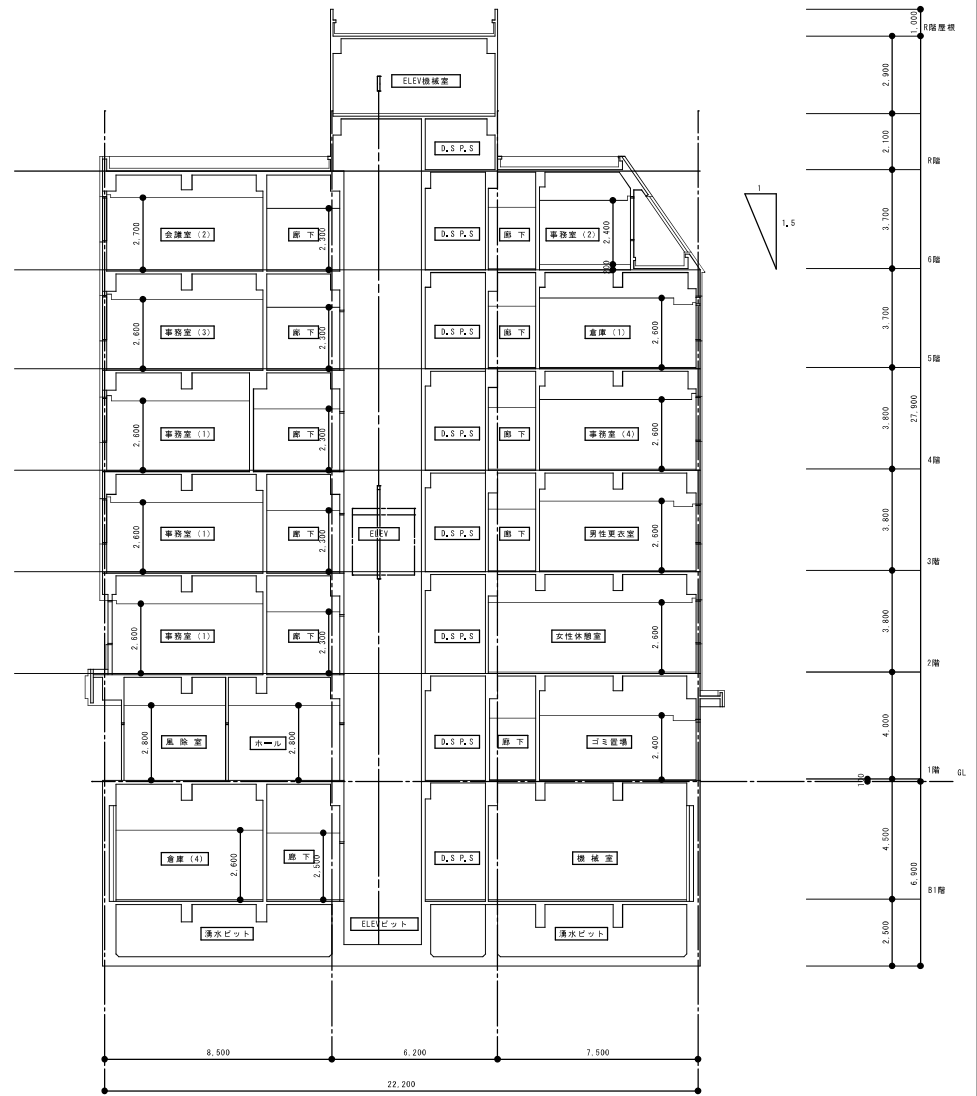
南一北断面図 1/200
