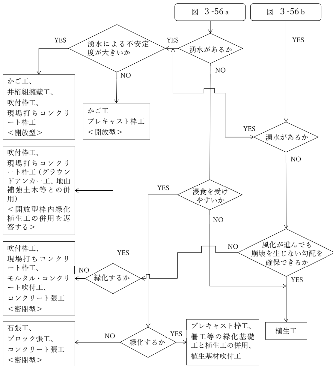
図 3-58 法面保護工の選定フロー③（切土法面の場合）[引用]道路土工 切土・斜面安定工指針（平成21年度版）、一部加工
