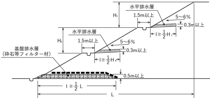
図 3-72 水平排水層
