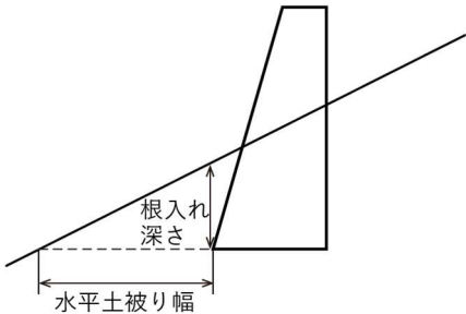
図 3-45 水平土被り
