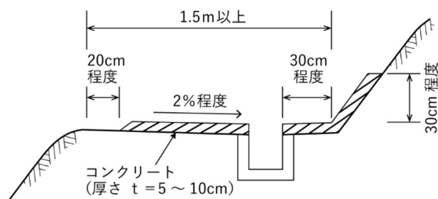
図 3-64 小段排水工
