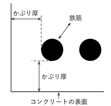
図 3-26 鉄筋のかぶり厚さ
