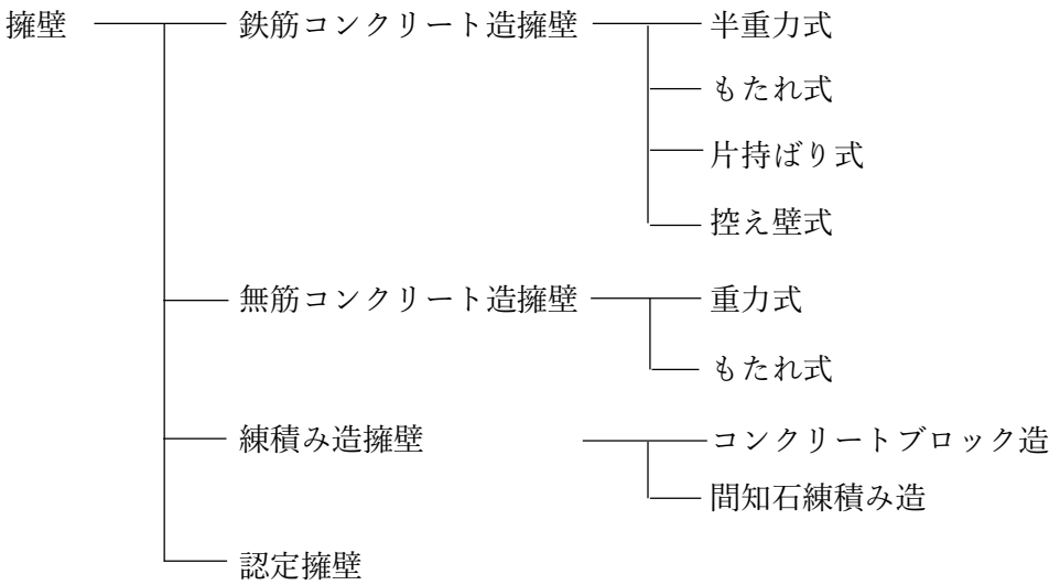
図 3-11 擁壁の種類
