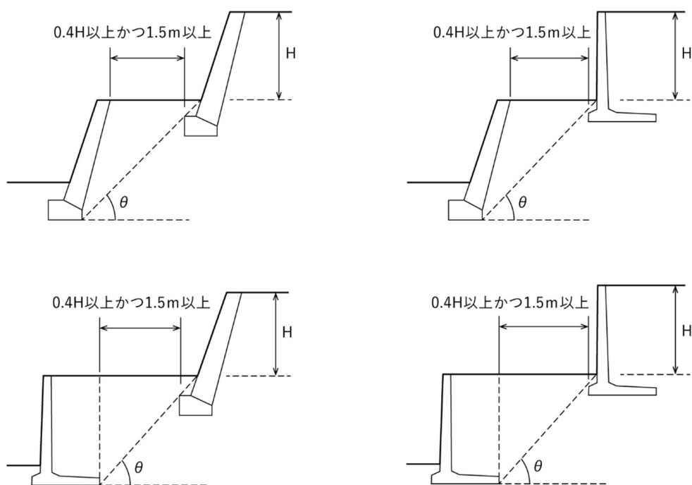
図 3-15 上部・下部擁壁を近接して設置する場合の考え方
