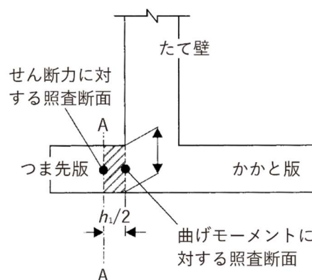
図 3-41 つま先版のせん断力を照査する断面
