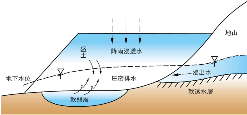
図 3-66 地下水の各構成成分
