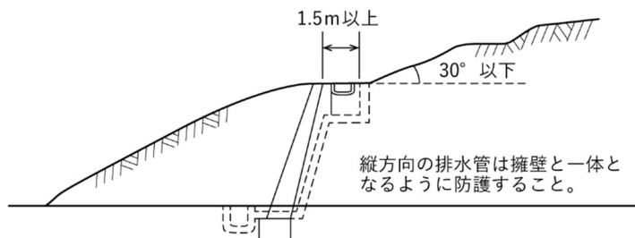
図 3-63 法肩排水工
