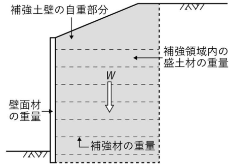
図 3-47 補強土壁の自重の考え方（安定性の照査時）
