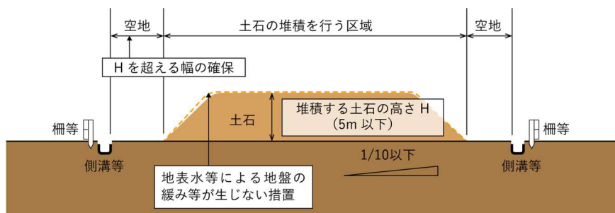
図 3-74 堆積する土地の基準（高さ 5m 以下）
