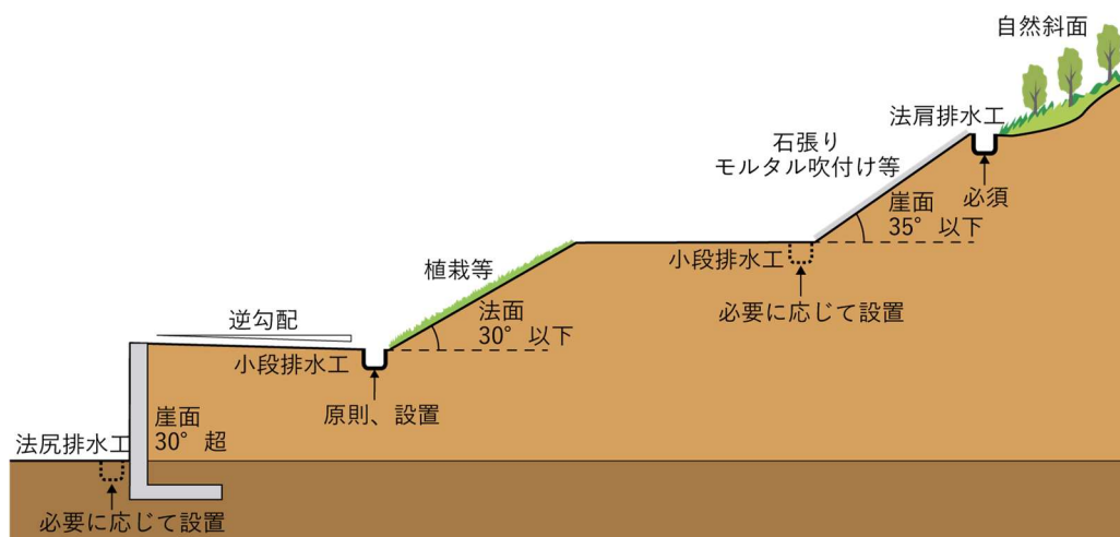
図 3-62 表面排水工の配置
