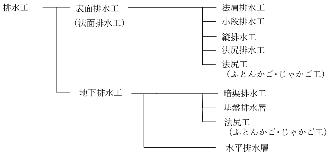
図 3-59 排水工の分類
