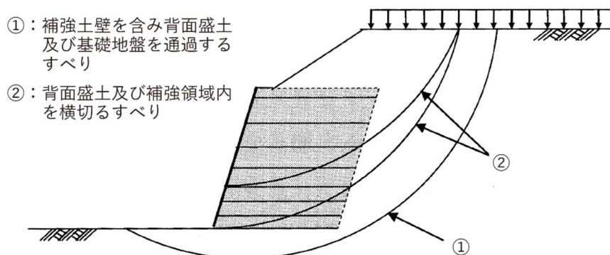
図 3-46 想定される全てのすべり面に対する安定の照査
