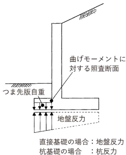
図 3-40 つま先版に作用する荷重
