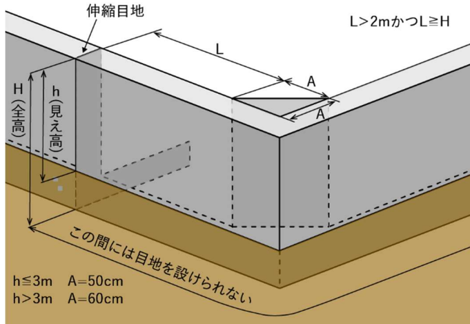
図 3-22 鉄筋コンクリート造擁壁等の伸縮目地及び隅角部の補強位置①
