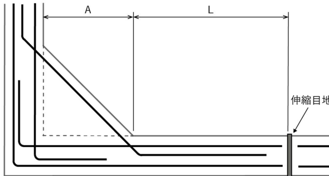
図 3-23 鉄筋コンクリート造擁壁等の伸縮目地及び隅角部の補強位置②
