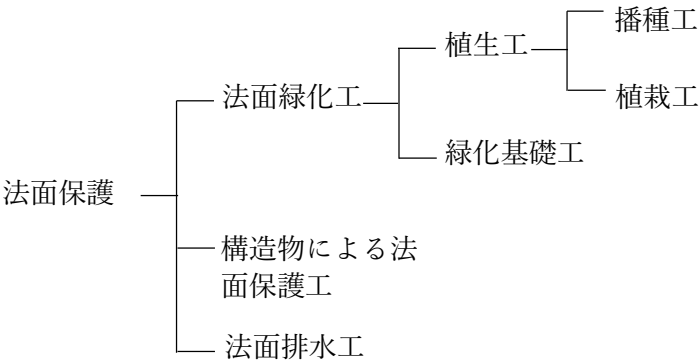
図 3-53 法面保護工の分類
