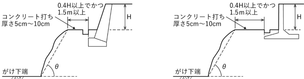
図 3-14 斜面の擁壁の構造
