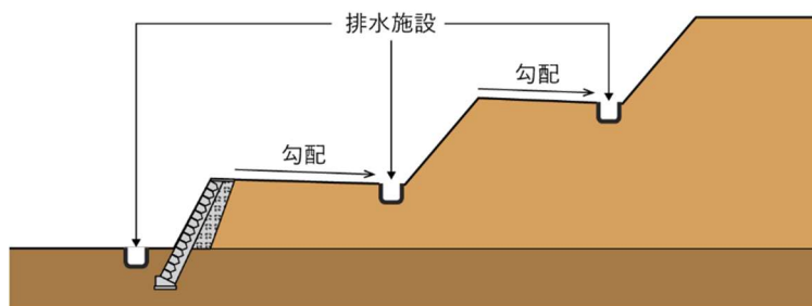
図 3-54 崖面天端の勾配
