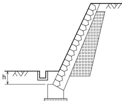
図 3-18 U 字溝に接する場合の根入れ
