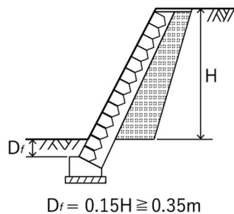
図 3-16 根入れ深さの考え方
