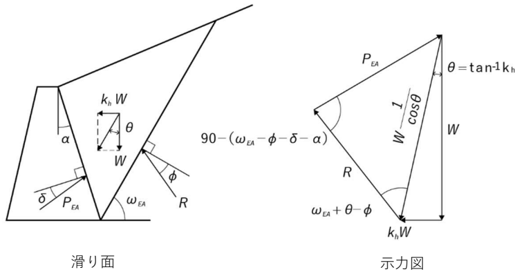
図 3-33 地震時主働土圧の考え方
