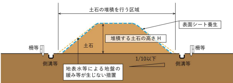
図 3-78 防水性シート等による保護
