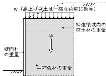
図 3-48 補強土壁の自重の考え方（部材の安全性の照査時）
