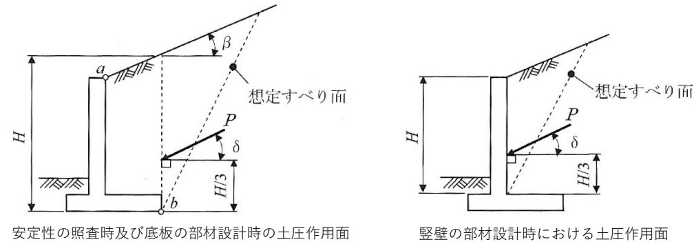
図 3-30 土圧作用面（片持ばり式）
