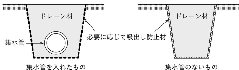
図 3-67 地下排水工の断面
