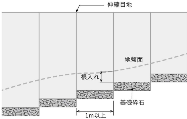
図 3-13 斜面に沿って設置する擁壁
