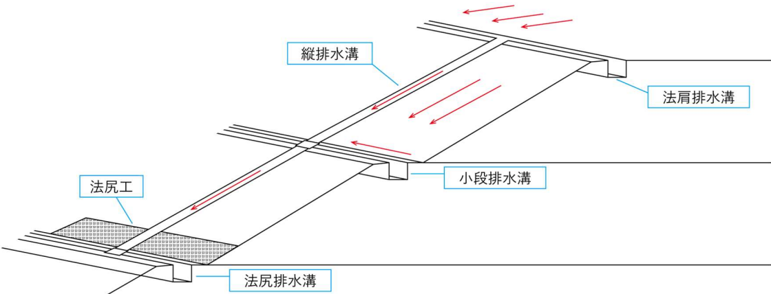
図 3-61 表面排水工の種類
