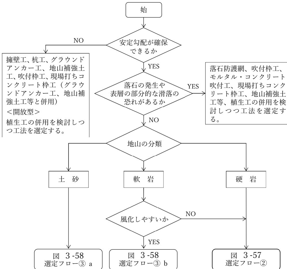
図 3-56 法面保護工の選定フロー①（切土法面の場合）
