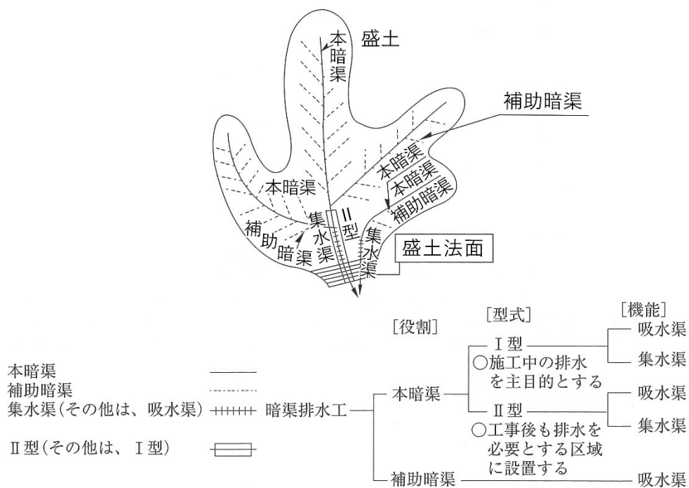
図 3-68 地下水排水工の配置
