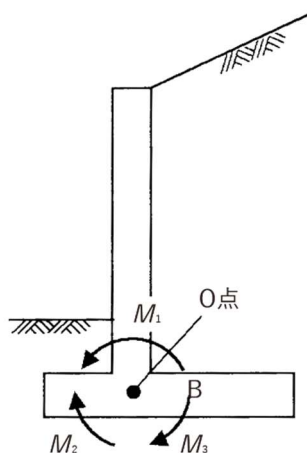
図 3-44 曲げモーメントの関係
