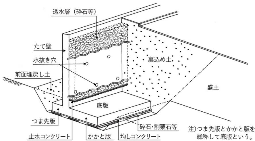
図 3-12 擁壁各部の名称
