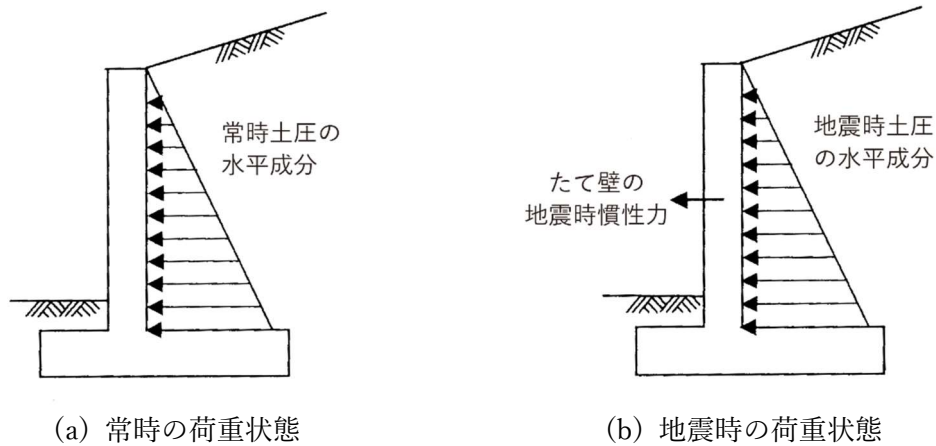
図 3-39 縦壁の断面計算における荷重状態
