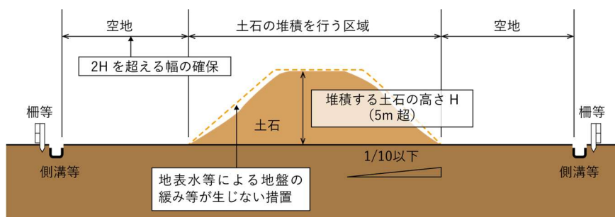
図 3-75 堆積する土地の基準（高さ 5m 超）
