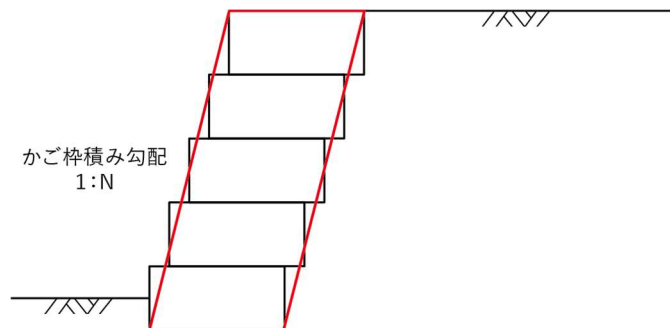
図 3-51 仮想断面の設定
