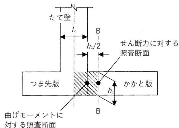
図 3-43 かかと版のせん断力を照査する断面
