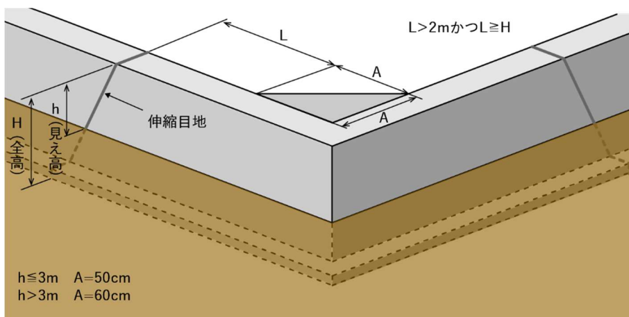
図 3-24 練積み造擁壁の伸縮目地及び隅角部の補強位置
