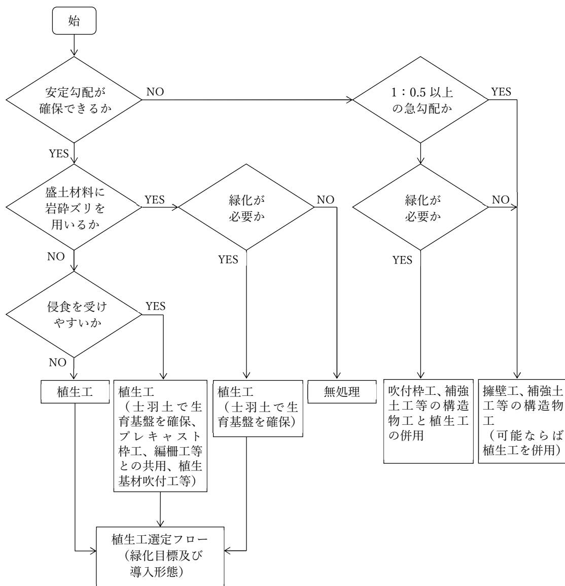
図 3-55 法面保護工選定フロー（盛土法面の場合）
