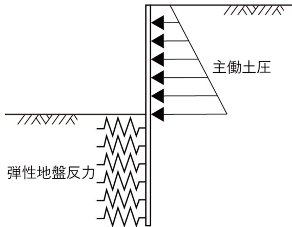
図 3-80 簡便法の計算モデル (Chang の式による)
