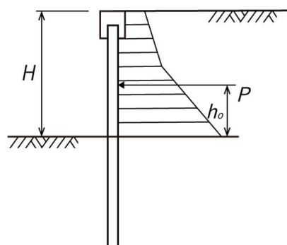
図 3-81 鋼矢板擁壁に作用する土圧及び水圧
