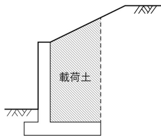
図 3-28 載荷土
