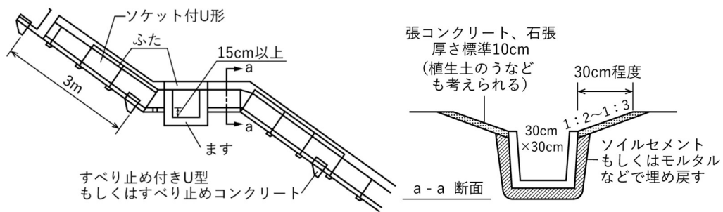
図 3-65 U型による縦排水工の構造図
