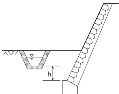
図 3-17 水路に近接する場合の根入れ
