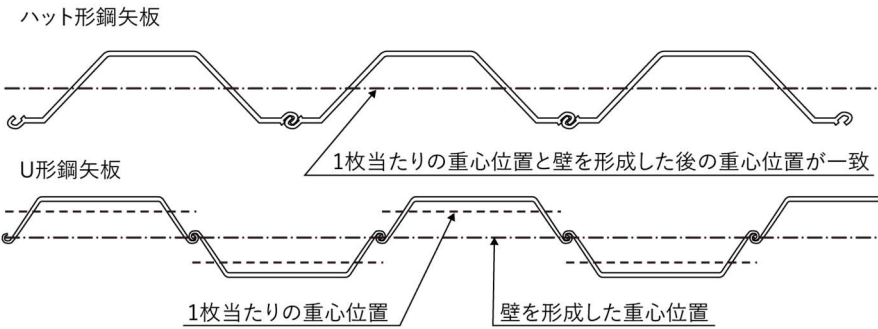
図 3-79 鋼矢板の単体と壁体の重心位置の関係
