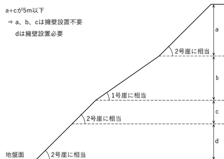
図 3-10 上下に分離された崖の部分がある場合の考え方
