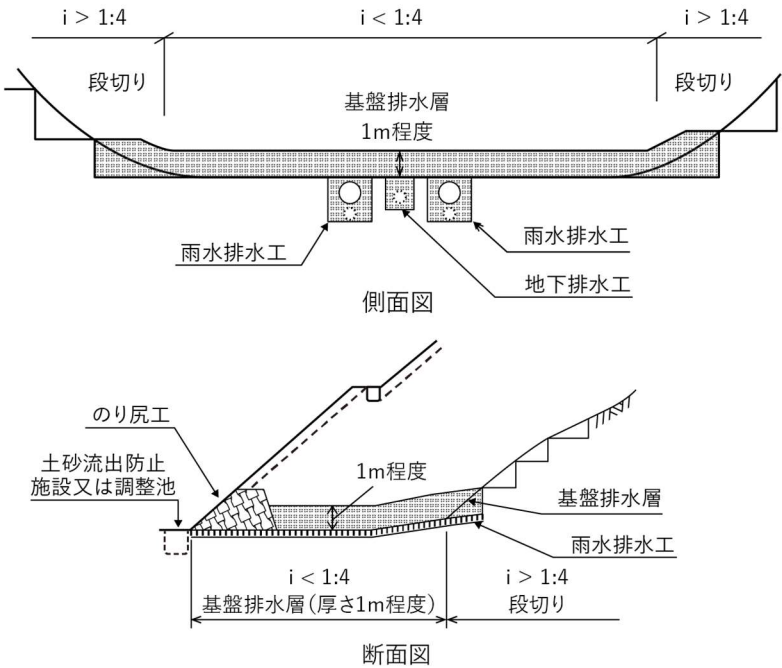
図 3-69 基盤排水層
