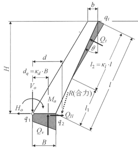
圖 3-38 地盤反力係數法 (簡便法)
