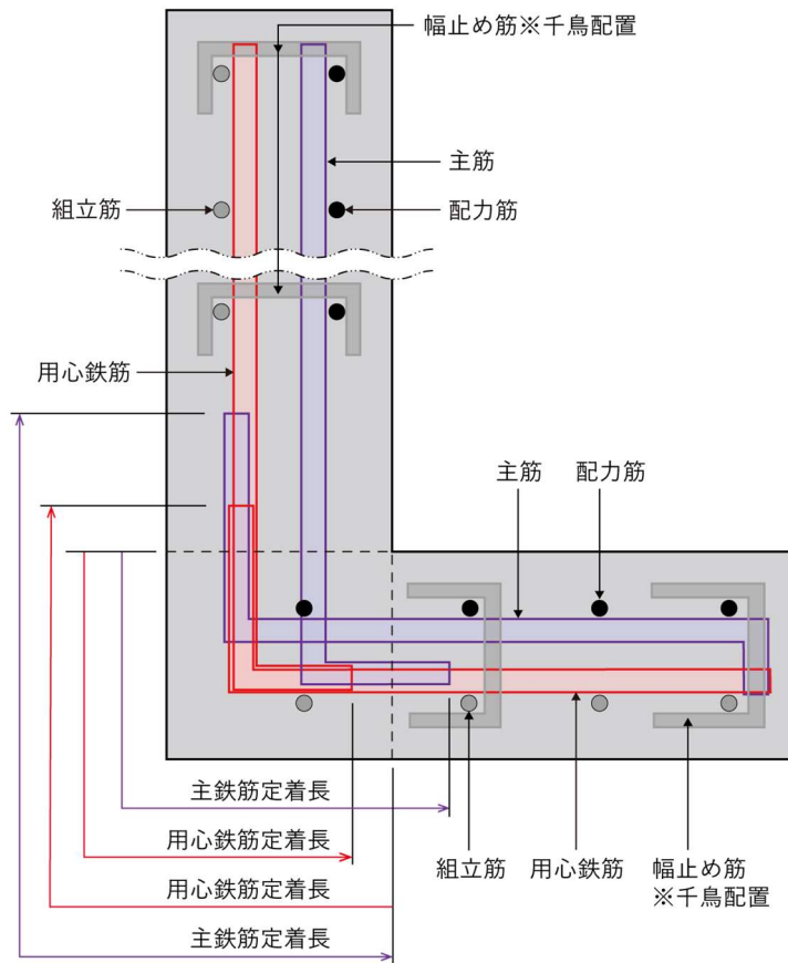
図 3-27 L型鉄筋コンクリート擁壁縦壁基部の配筋要領
