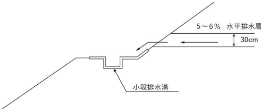
図 3-71 水平排水層端末部
