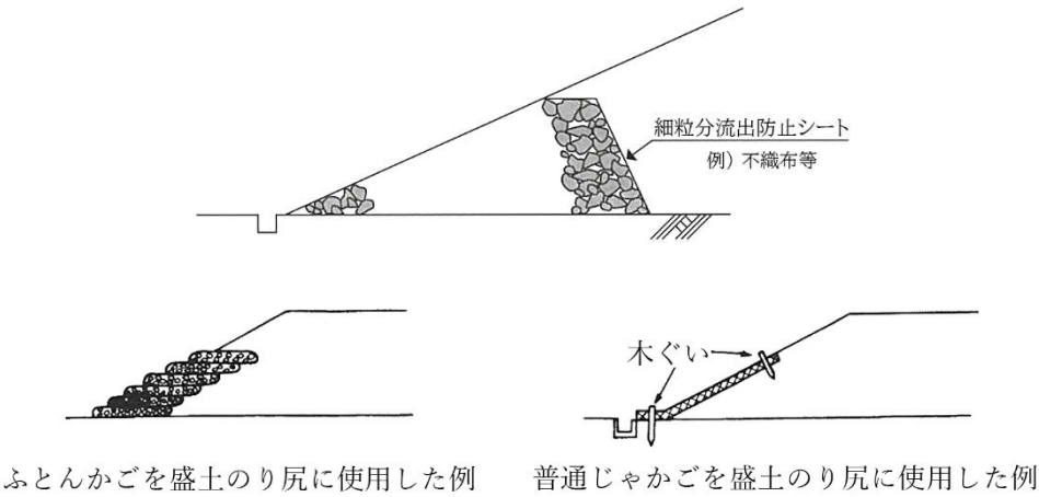
図 3-70 法尻工の例
