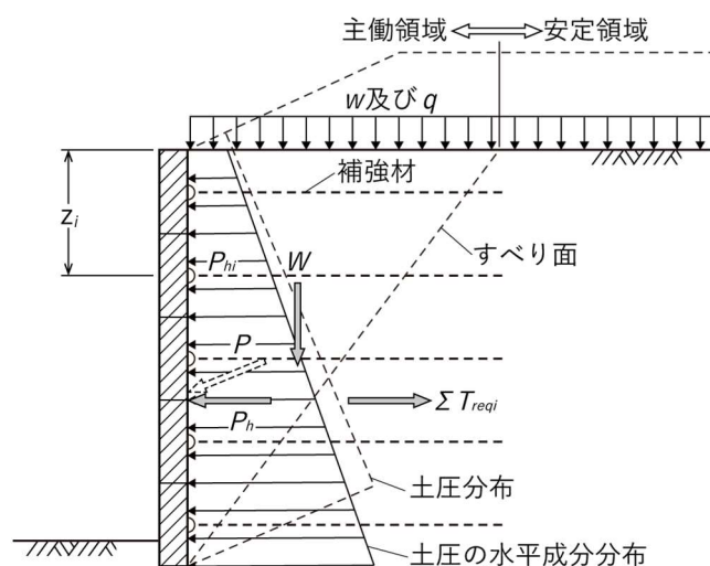
図 3-49 補強土壁自体の安定性の照査に用いる土圧
