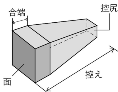
図 3-19 間知ブロックの各部名称
