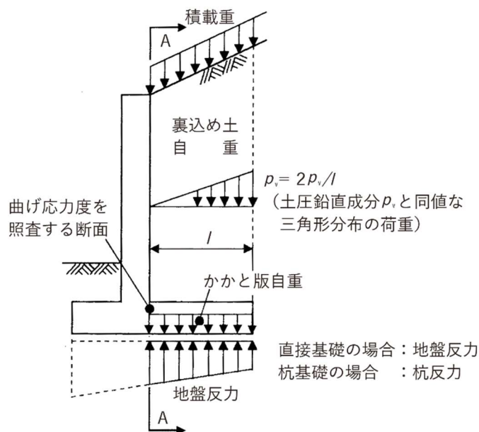
図 3-42 かかと版に作用する荷重
