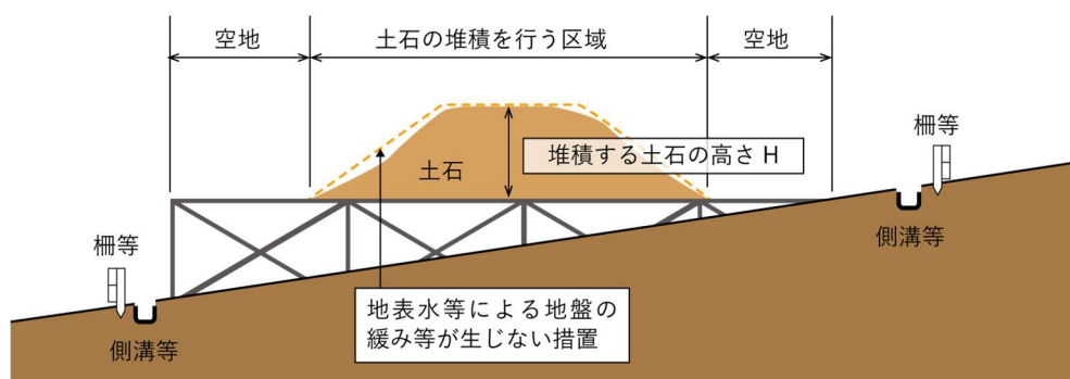
図 3-76 構台のイメージ
