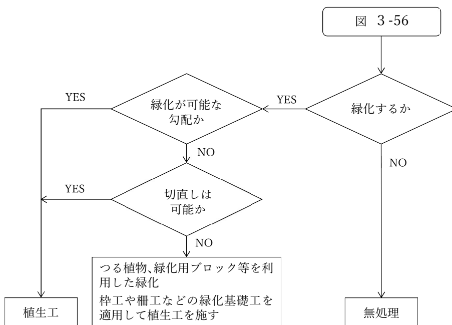
図 3-57 法面保護工の選定フロー②（切土法面の場合）
