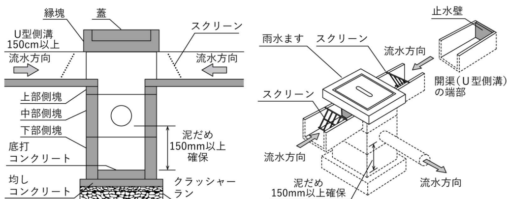
図 3-60 排水工の標準構造図
