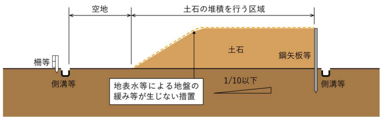
図 3-77 鋼矢板等の設置
