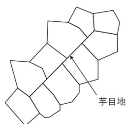
図 4-5 芋目地の組積みの例（施工してはならない積み方）
