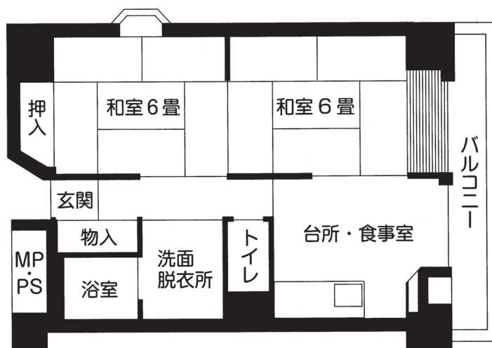
A タイプ 2DK (52.01m²)
