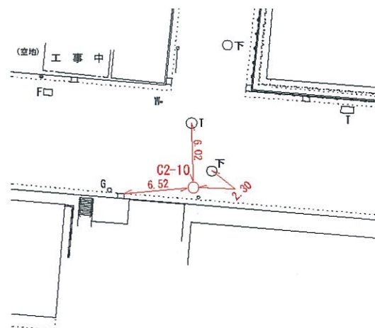
詳細図
