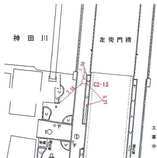
詳細図
