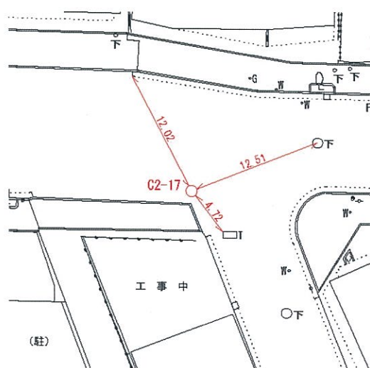
詳細図
