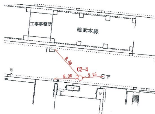
詳細図
