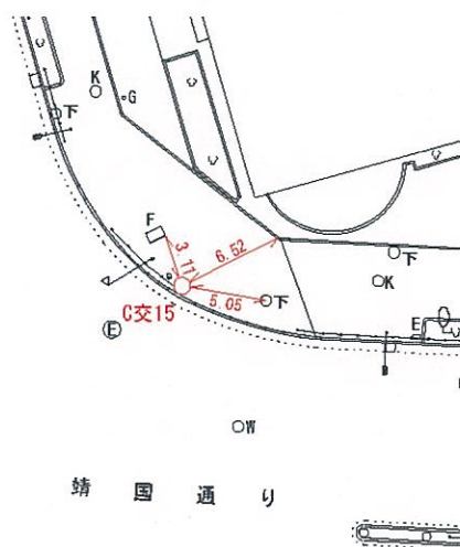
詳細図
