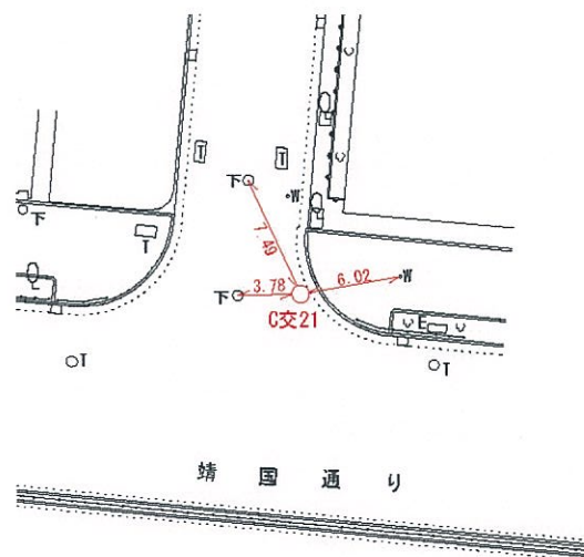
詳細図
