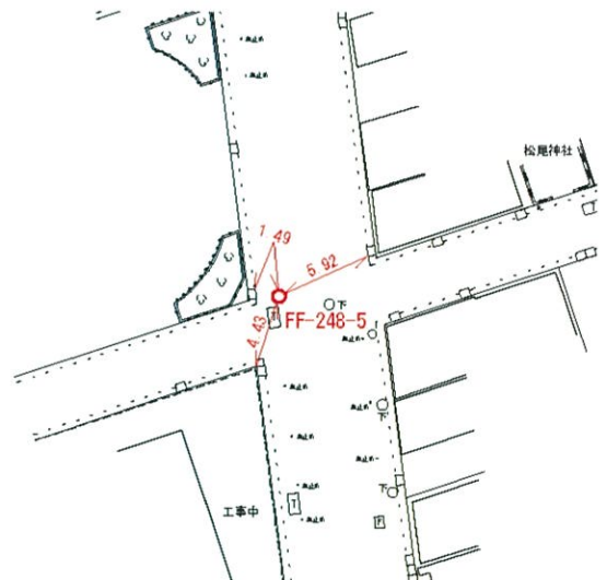
詳細図
