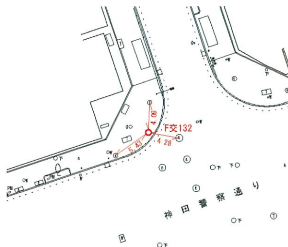
詳細図
