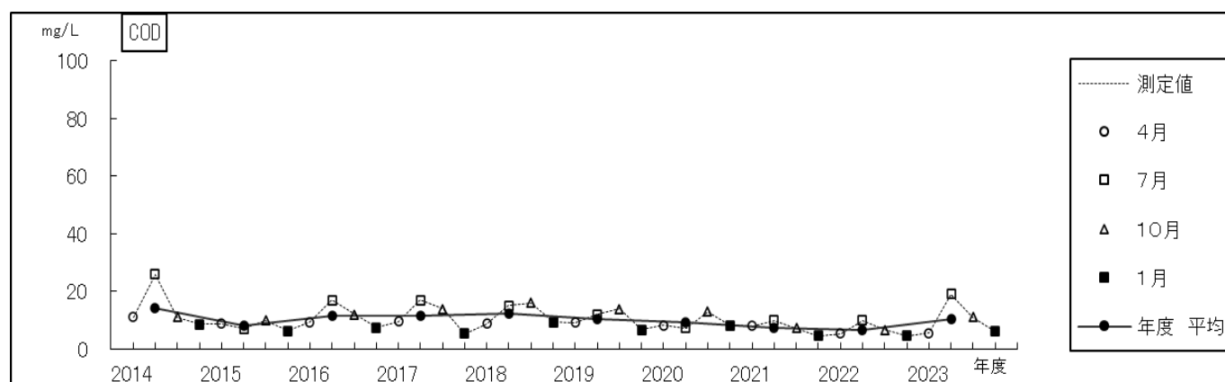
過去10年間の経年変化（化学的酸素要求量一千鳥ヶ淵）
