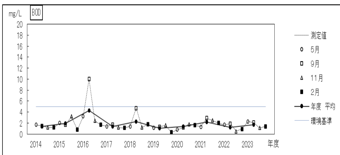
過去10年間の経年変化(生物化学的酸素要求量－常盤橋)
