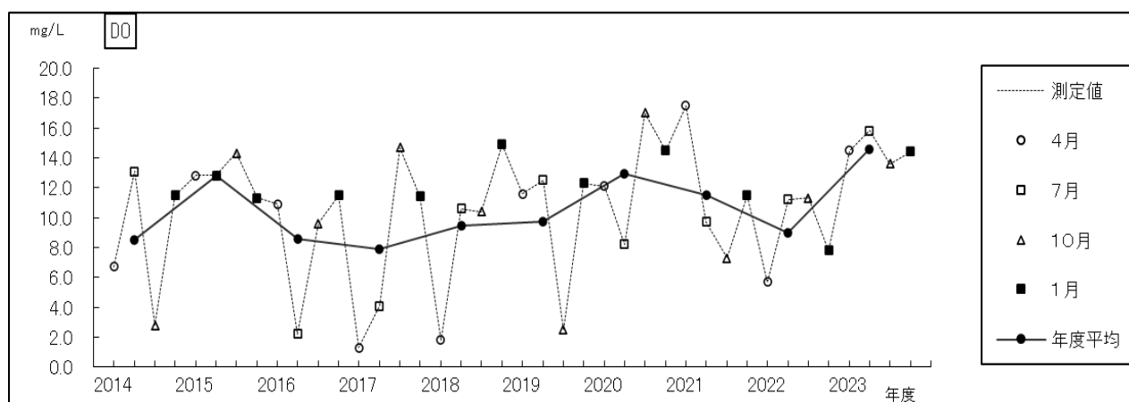
過去10年間の経年変化(溶存酸素－市ヶ谷濠)
