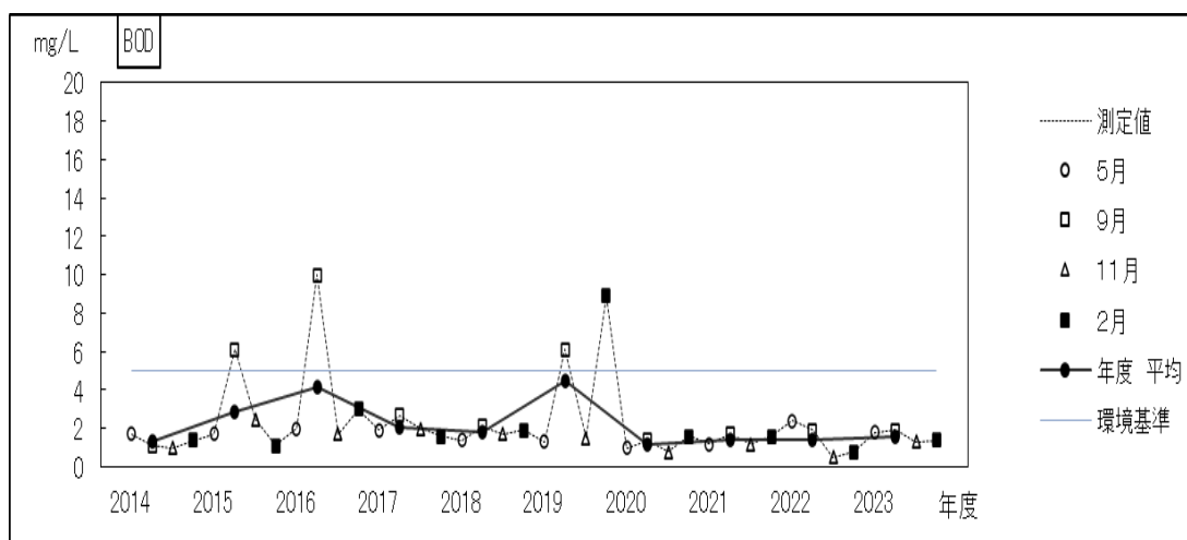
過去10年間の経年変化(生物化学的酸素要求量－堀留橋)
