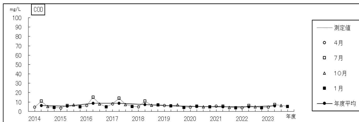
過去10年間の経年変化（化学的酸素要求量一日比谷濠）
