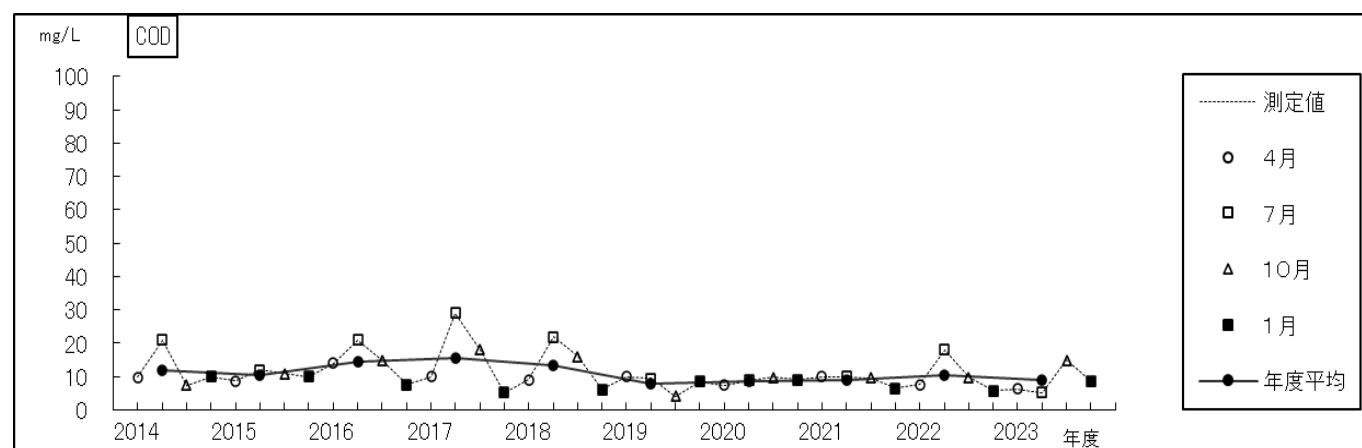
過去10年間の経年変化(化学的酸素要求量－新見附濠)
