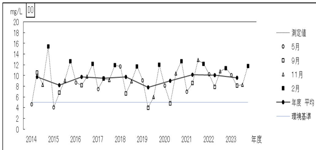
過去10年間の経年変化(溶存酸素－牛込橋)
