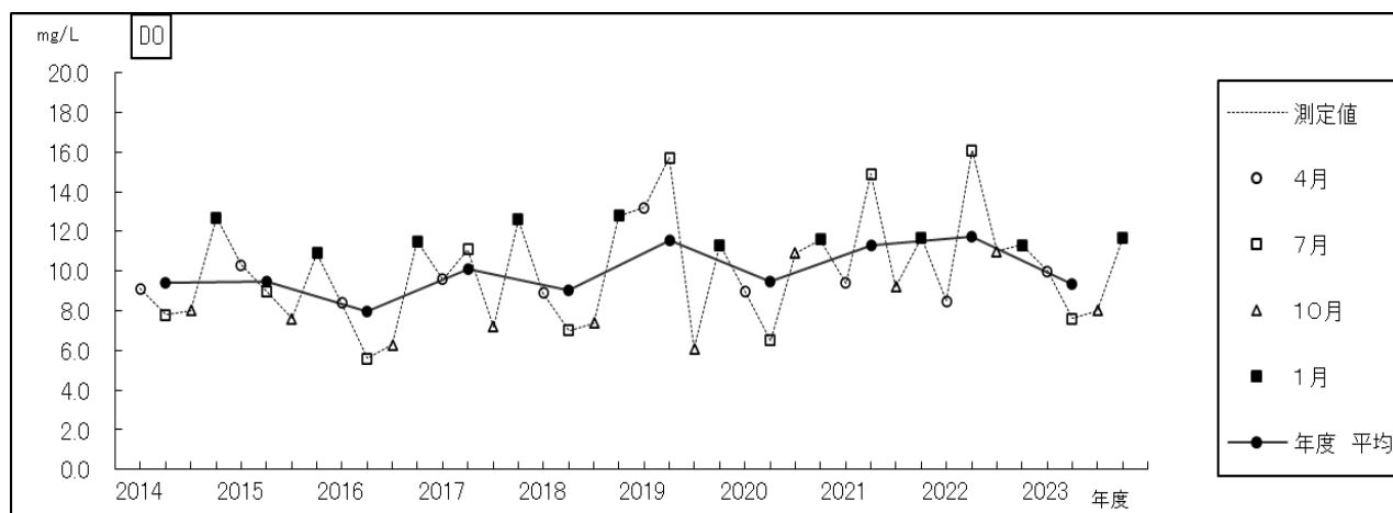
過去10年間の経年変化(溶存酸素－弁慶濠)
