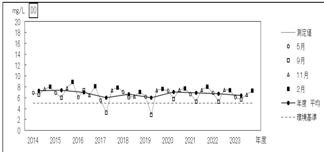
過去10年間の経年変化(溶存酸素－飯田橋)
