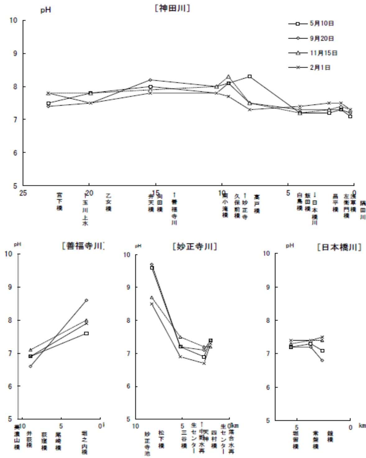
神田川流域 pH変化図 (2023年度)
