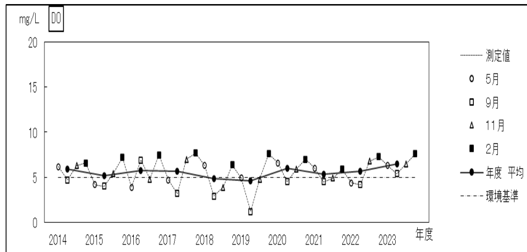
過去10年間の経年変化(溶存酸素－昌平橋)
