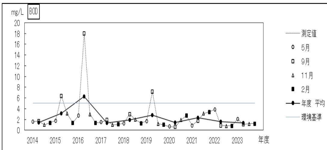
過去10年間の経年変化 (生物化学的酸素要求量－昌平橋)
