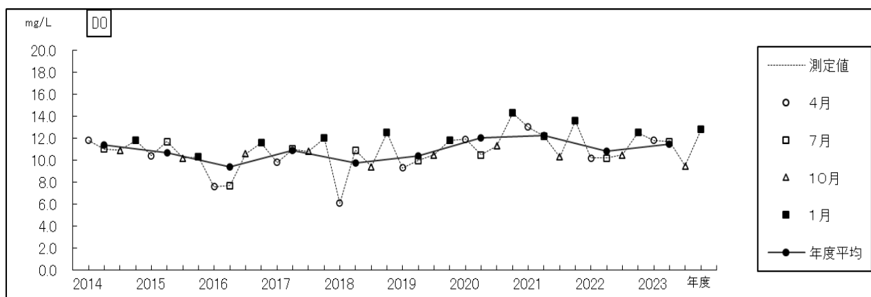
過去10年間の経年変化(溶存酸素－一日比谷濠)
