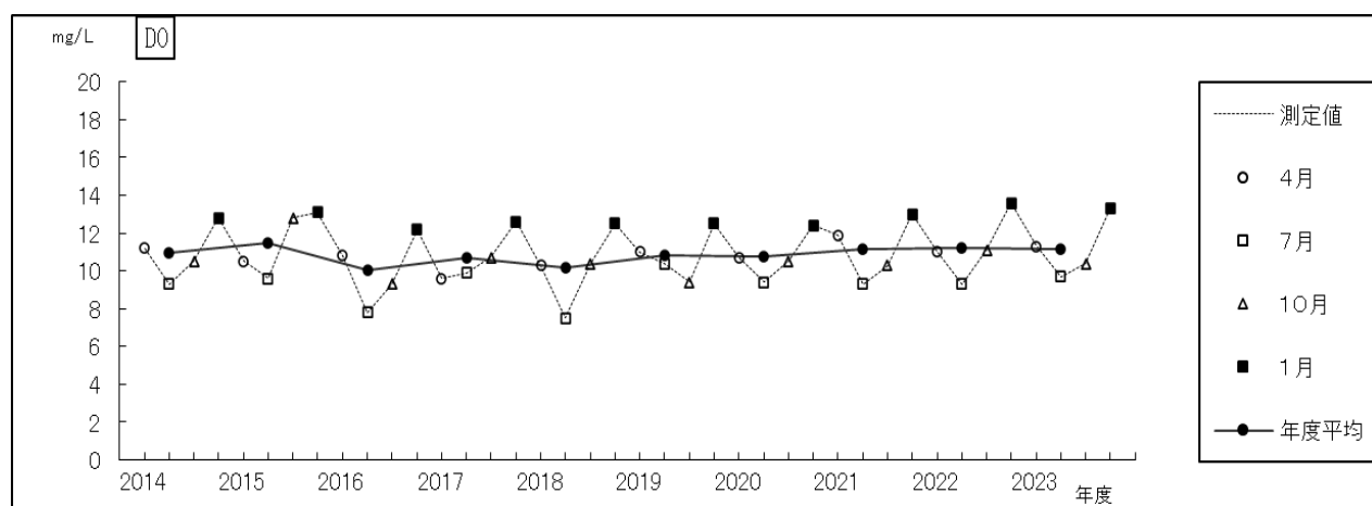
過去10年間の経年変化(溶存酸素－半蔵濠)
