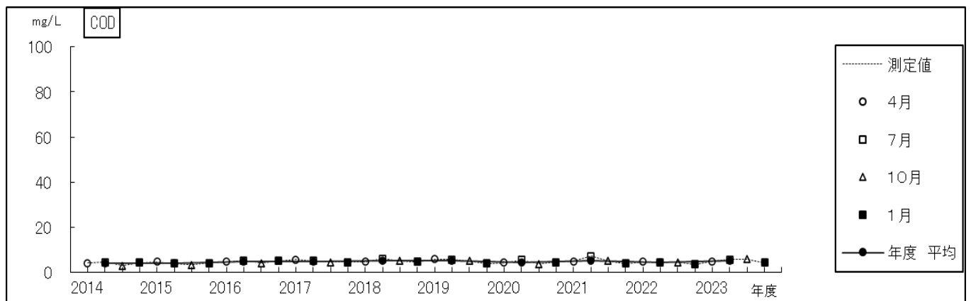
過去10年間の経年変化(化学的酸素要求量一弁慶濠)
