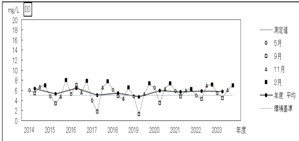
過去10年間の経年変化(溶存酸素－堀留橋)
