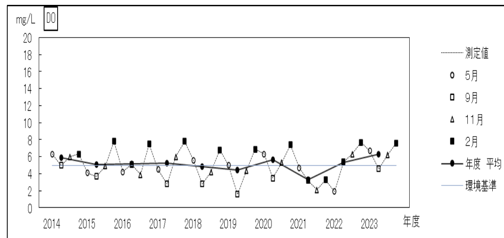
過去10年間の経年変化(溶存酸素－左衛門橋)
