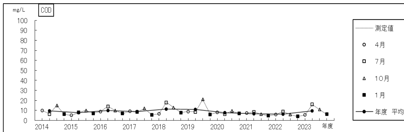
過去10年間の経年変化(化学的酸素要求量－牛ヶ淵)
