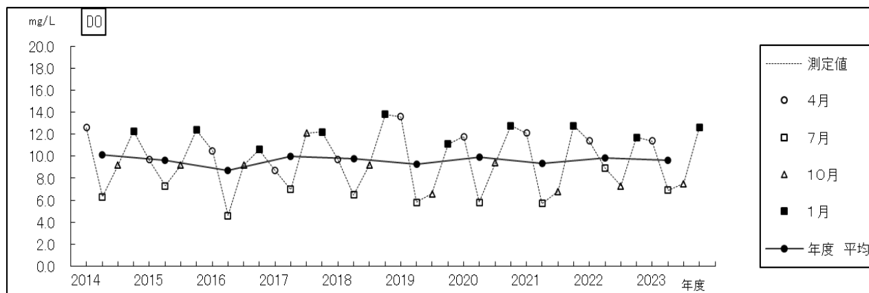
過去10年間の経年変化(溶存酸素－牛ヶ淵)
