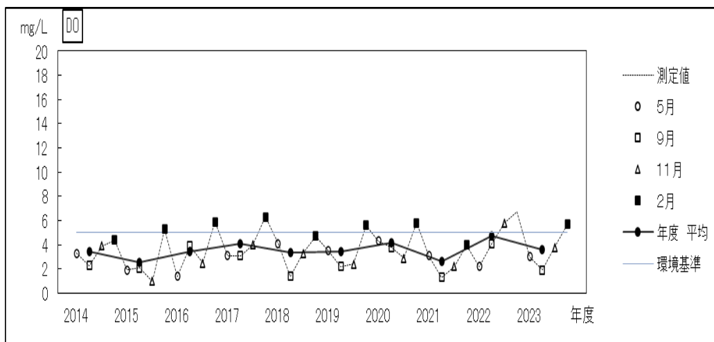
過去10年間の経年変化(溶存酸素－常盤橋)
