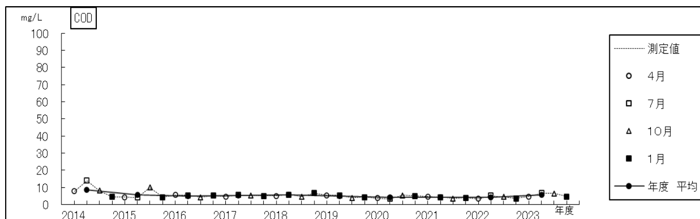
過去10年間の経年変化（化学的酸素要求量一半蔵濠）
