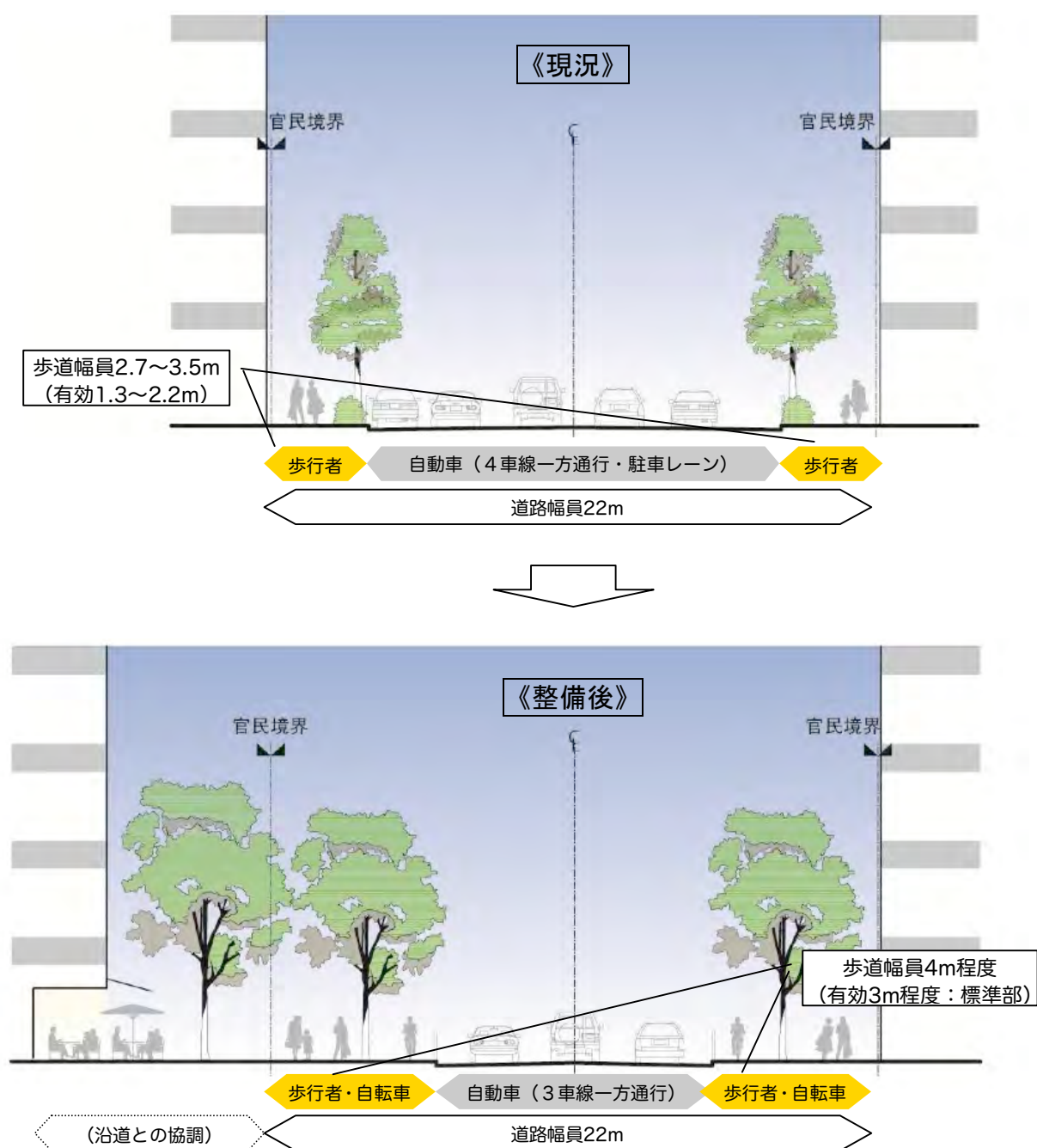
神田警察通りの整備イメージ（断面）
