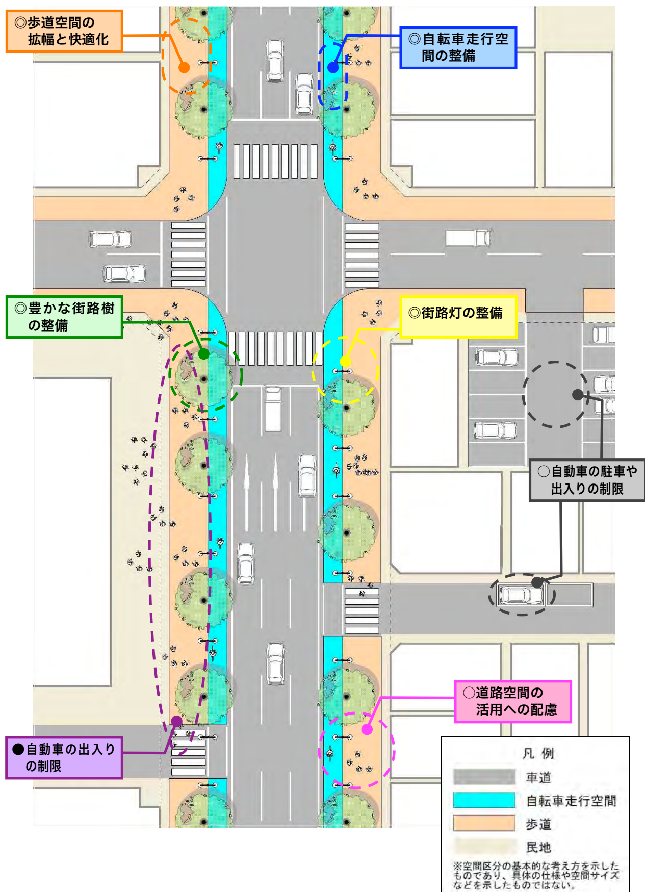
神田警察通りの整備イメージ（平面）
